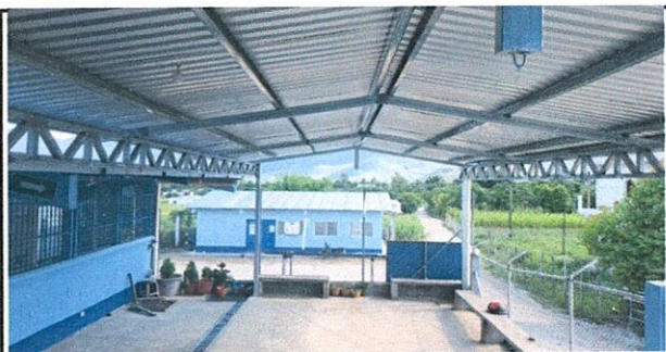
Foto 5: Suministro e instalación de estructura metálica para galera de 7.00 x 12.00 m, conformado por columna de tubo cuadrado, vigas principales y costaneras tipo lámina "YOS", incluyendo correas y herrajes de anclaje.
